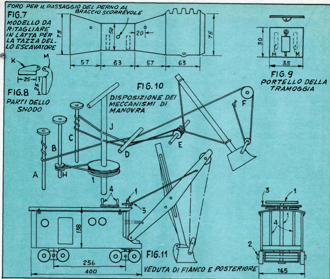
Dettagli completi, interni ed esterni, di un altro tipo di escavatrice. Nulla impedisce che qualche dettaglio di questa possa essere inserito in una delle quattro precedentemente illustrate.
