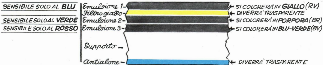
Fig. 4 - SEZIONE DI UNA PELLICOLA FERRANICOLOR, AGFACOLOR ECC.
